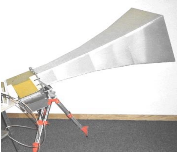
EMAG L-band Horn Antenna
